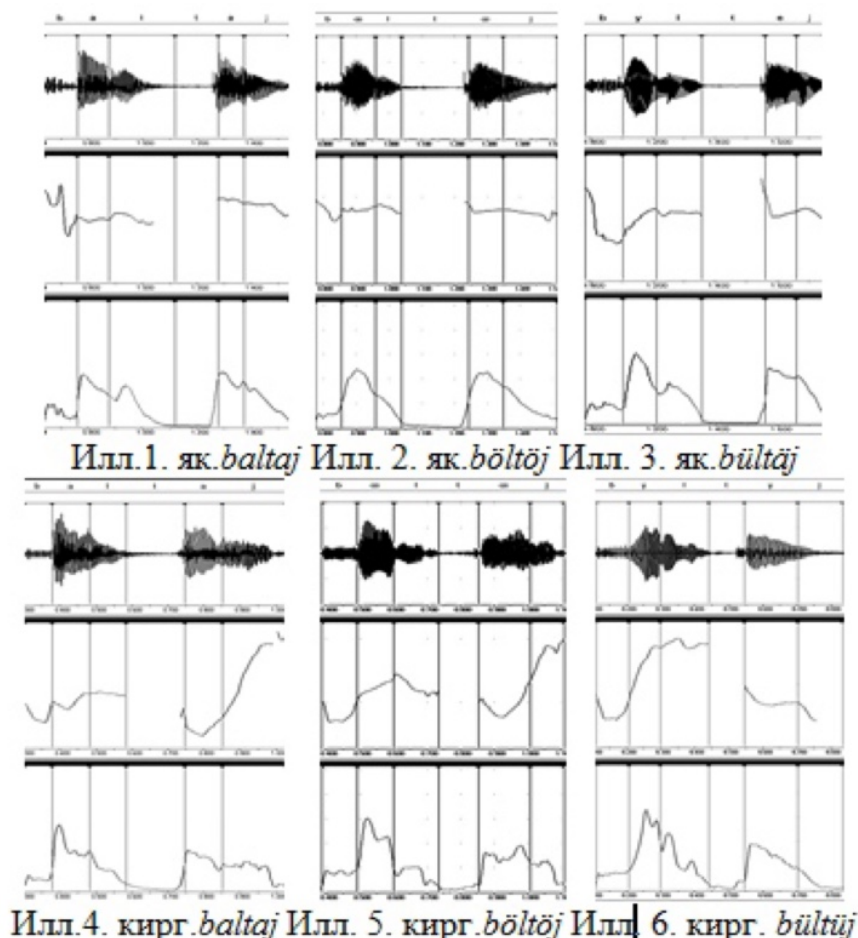
Рис. 1. Интонограммы
