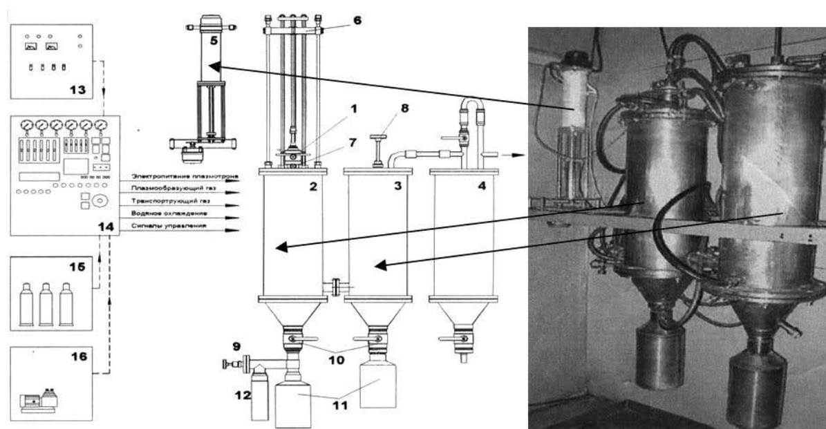
Рис. 3. Плазмохимическая установка конструкции ИМЕТ им. А.А. Байкова. 1– электродуговой плазматрон; 2–реактор; 3–аппарат фильтрации; 4–аппарат очистки отходящих газов; 5–дозатор порошковых материалов; 6–10–система удаления порошка из реактора; 11 – 12
